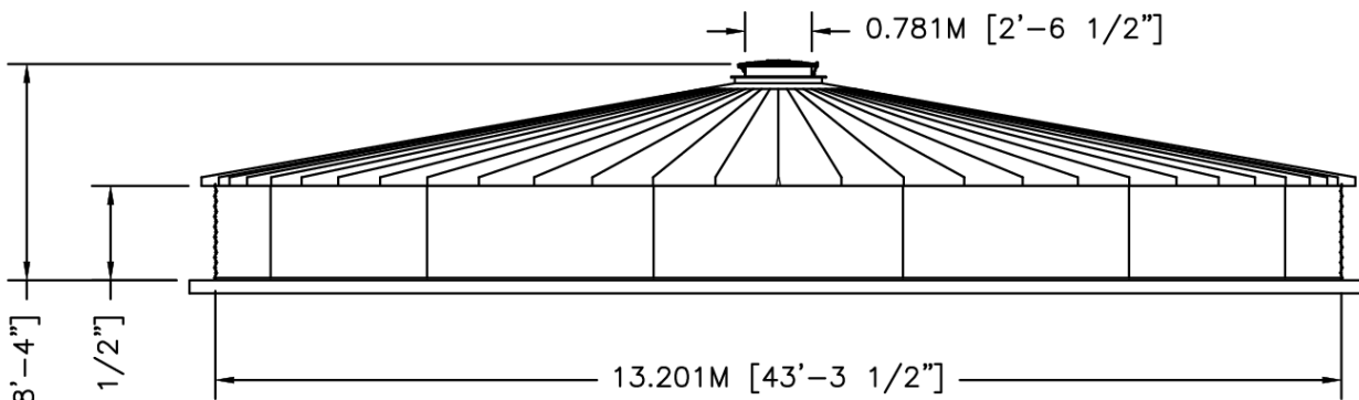
ELEVATION
