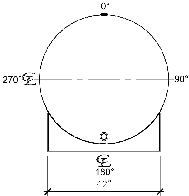
LEFT SIDE
