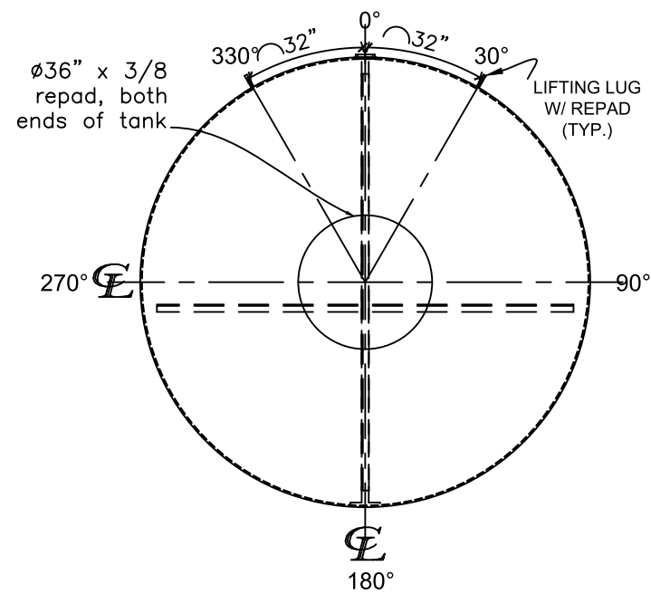
LEFT SIDE
